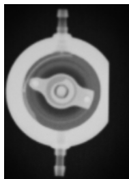
Fig. 18: Cliché radiologique, position 0 cmH 2 O
