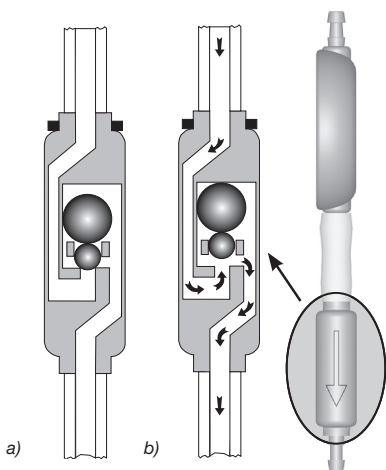
Abb. 5: Gravitationseinheit in aufrechter Körperhaltung
