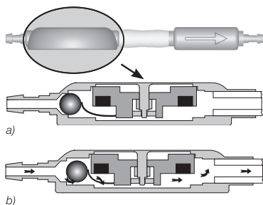
Abb. 4: Verstellbare Differenzdruckeinheit
