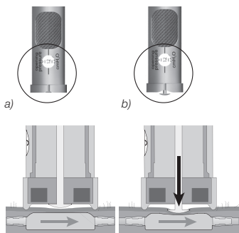
Fig. 15: Cambio de la presión de apertura de la válvula
