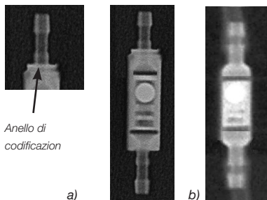
Fig. 7: Radiografia della valvola a gravitazione
