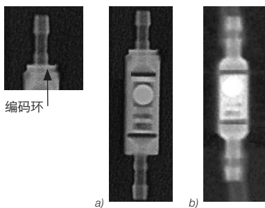
图7: 重力装置的X射线图像
