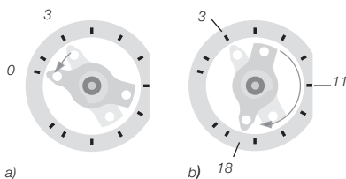
Fig. 16: Rotation du rotor lors du réglage
