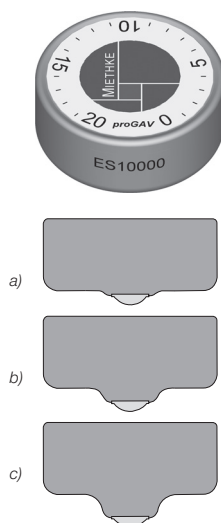
Abb. 10b: proGAV Verstelleiche
