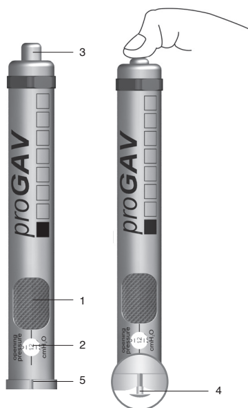
Abb. 10a: proGAV Verstellinstrument
