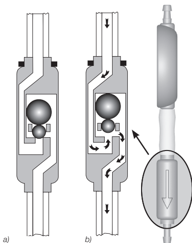
Fig. 5: Valvola a gravitazione in posizione eretta
