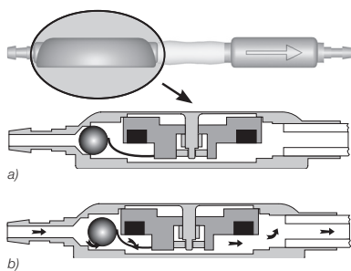
Fig. 4: Valvola a regolazione
