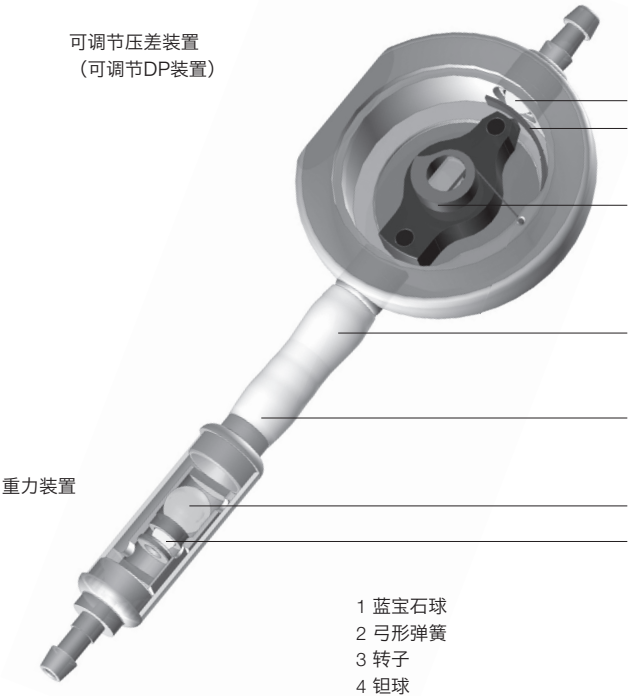
图2: proGAV 横截面示意图
