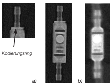
Abb. 7: Röntgenbild der Gravitationseinheit
